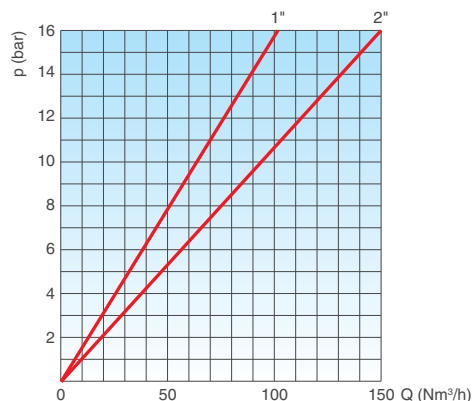
PURGA DE AIRE BAJO PRESIÓN
